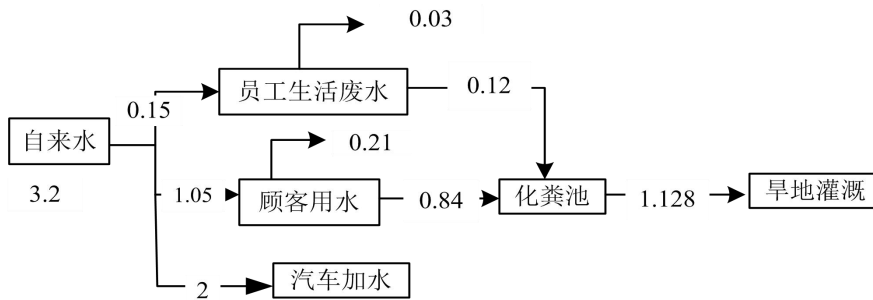
图 5.7 雨季水量平衡图 (单位: \text{m}^3/\text{d} )
