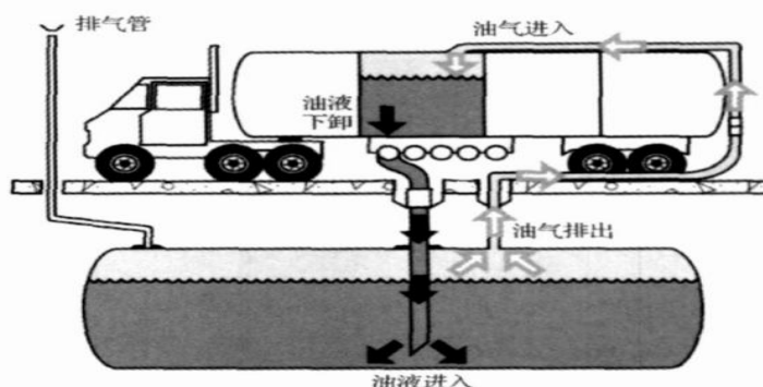
图 5.4 卸油过程回收系统示意图
